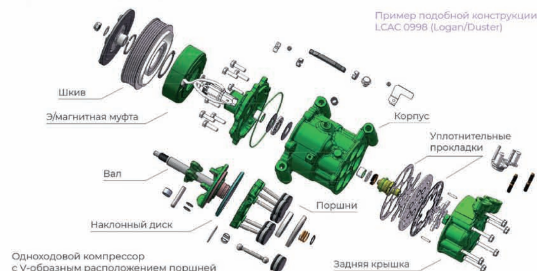
Схема 1 — поршневой компрессор
