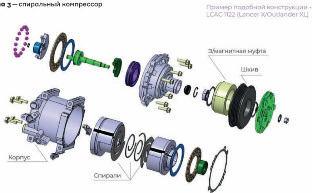
Схема 3 — спиральный компрессор
