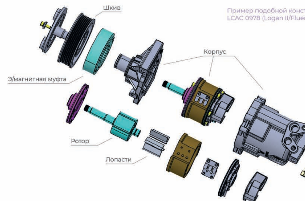
Схема 4 — роторно-лопастной компрессор
