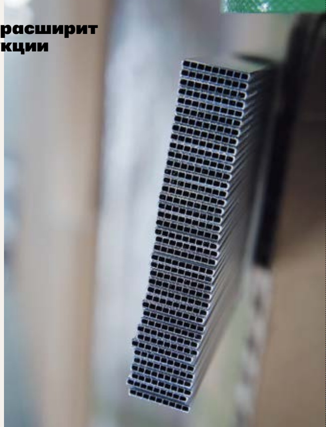
В конденсаторах MILES используются трубки со множеством внутренних каналов. Это улучшает процесс теплообмена
